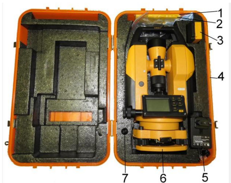
Рисунок 1 – Схема размещения в укладочном футляре
