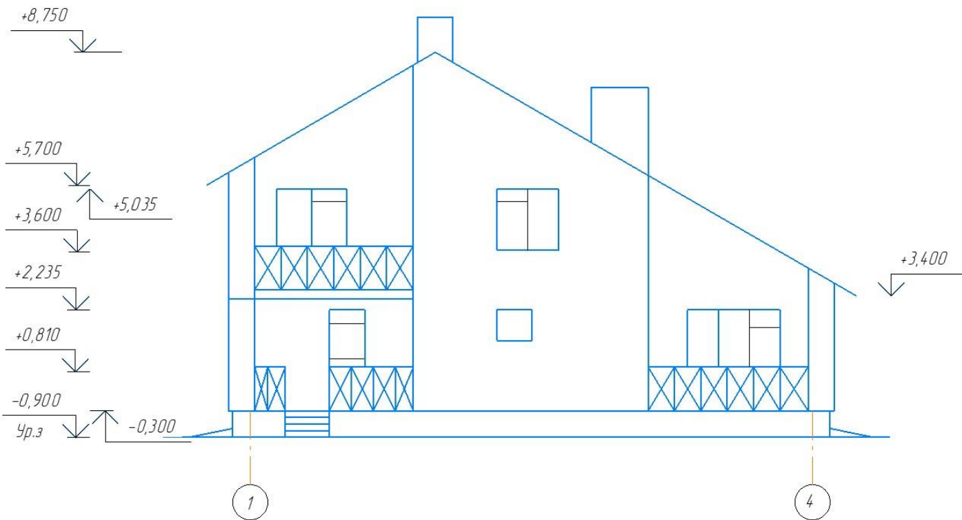
Фасад 1-4
