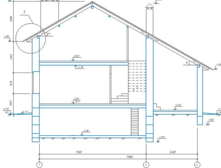
Разрез 1-1
