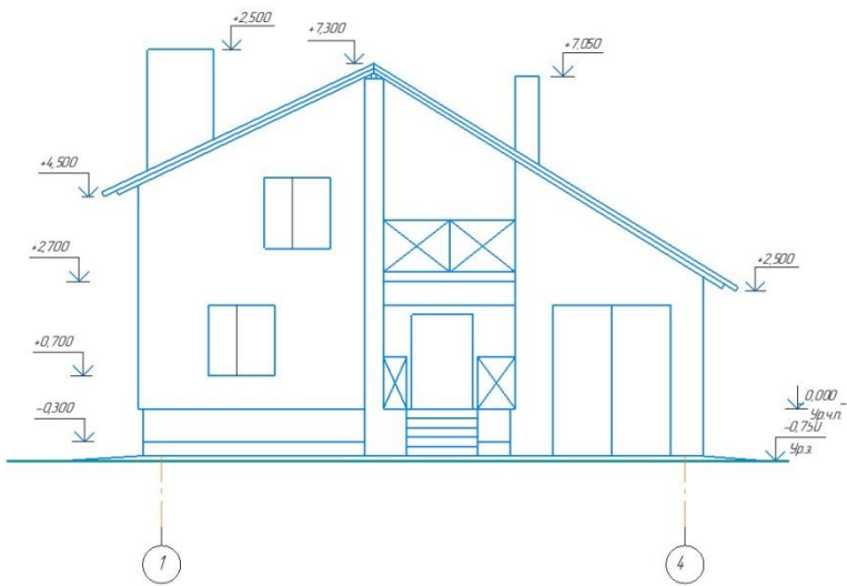
Фасад 1-4
