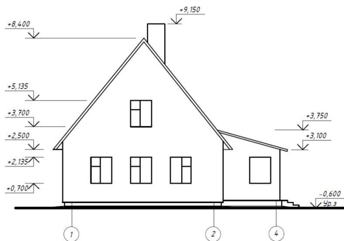
Фасад 1-4
