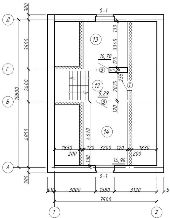
План мансарды
