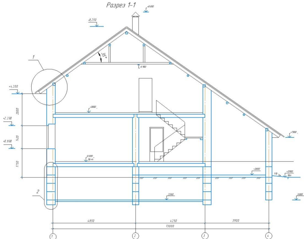
Разрез 1-1
