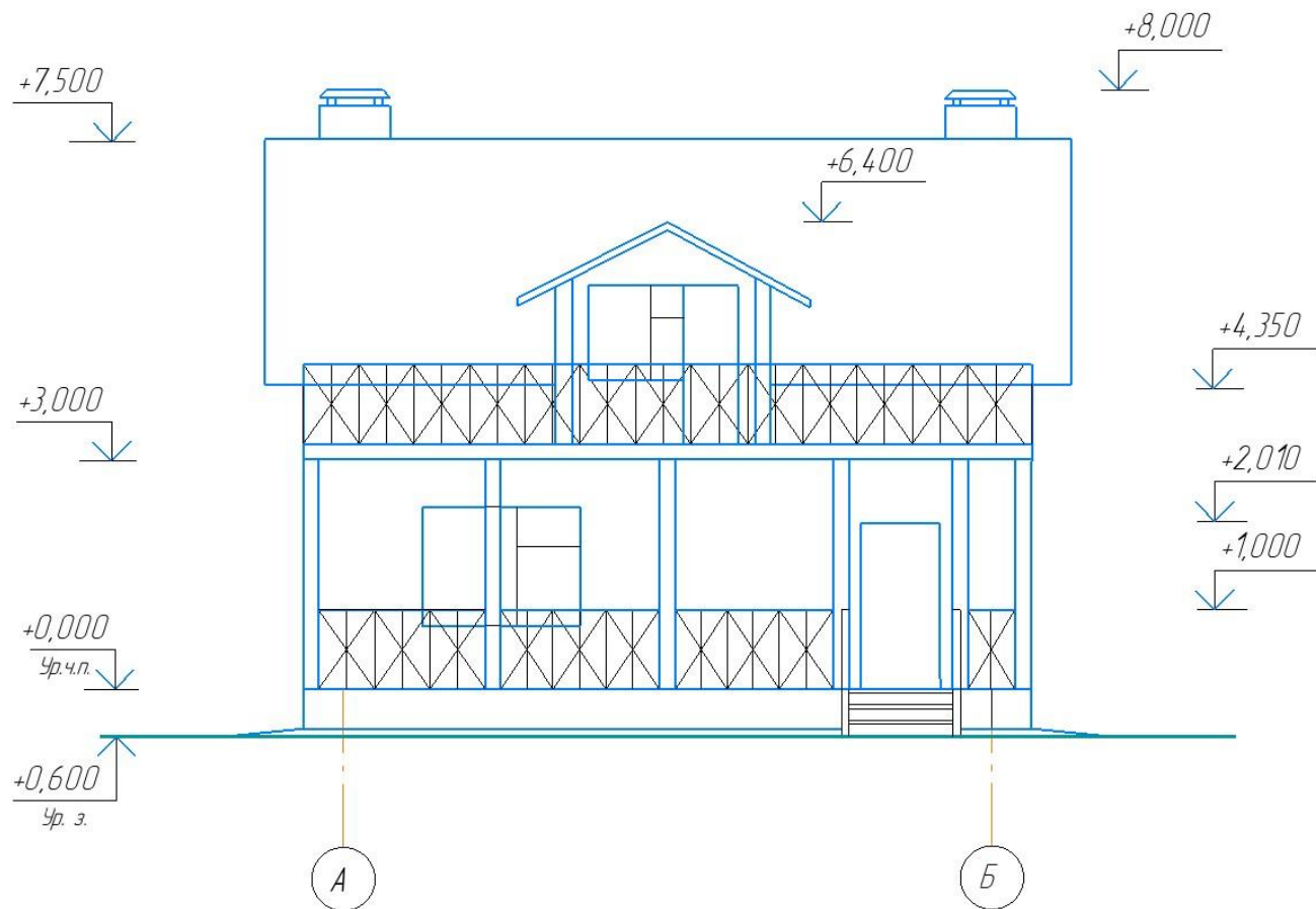
Фасад А-Б
