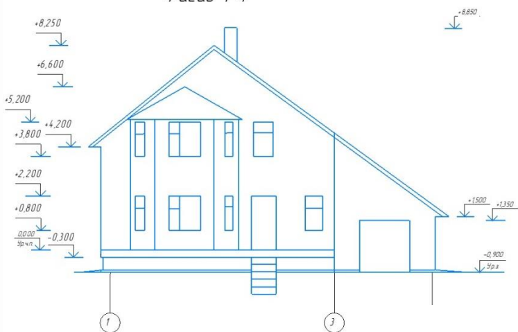
Фасад 1-4
