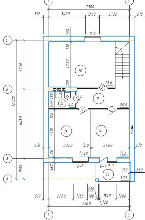
План мансарды
