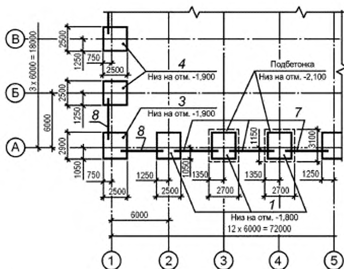
Рисунок Л.1 — Схема расположения элементов фундаментов и фундаментных блоков
